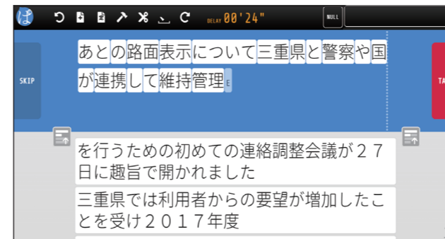
入力画面
