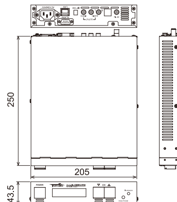
【外形図】
