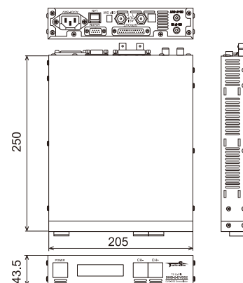
【外形図】
