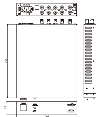
【外形図】
