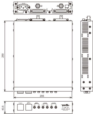
【外形図】
